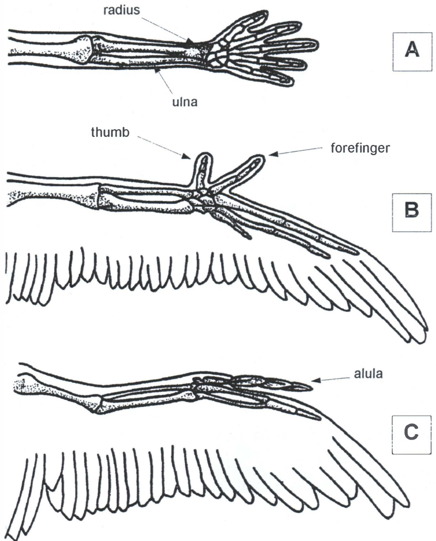
Abb. 3: Umwandlung eines humanen Vorderarmes in einen Vogelflügel A) früherer Mensch; B) als Zwischenstufe mögliche Gestaltung vom Flügel eines hypothetischen pro-Avis; C) Vogelflügel im Endstadium. Skizze: © de Sarre
