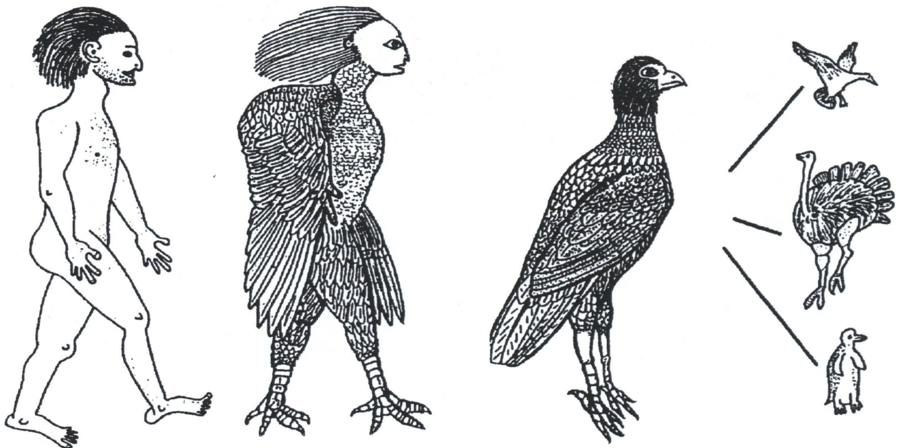
Abb. 5: Versuch einer phylogenetischen Rekonstruktion der Vogelreihe von links nach rechts
