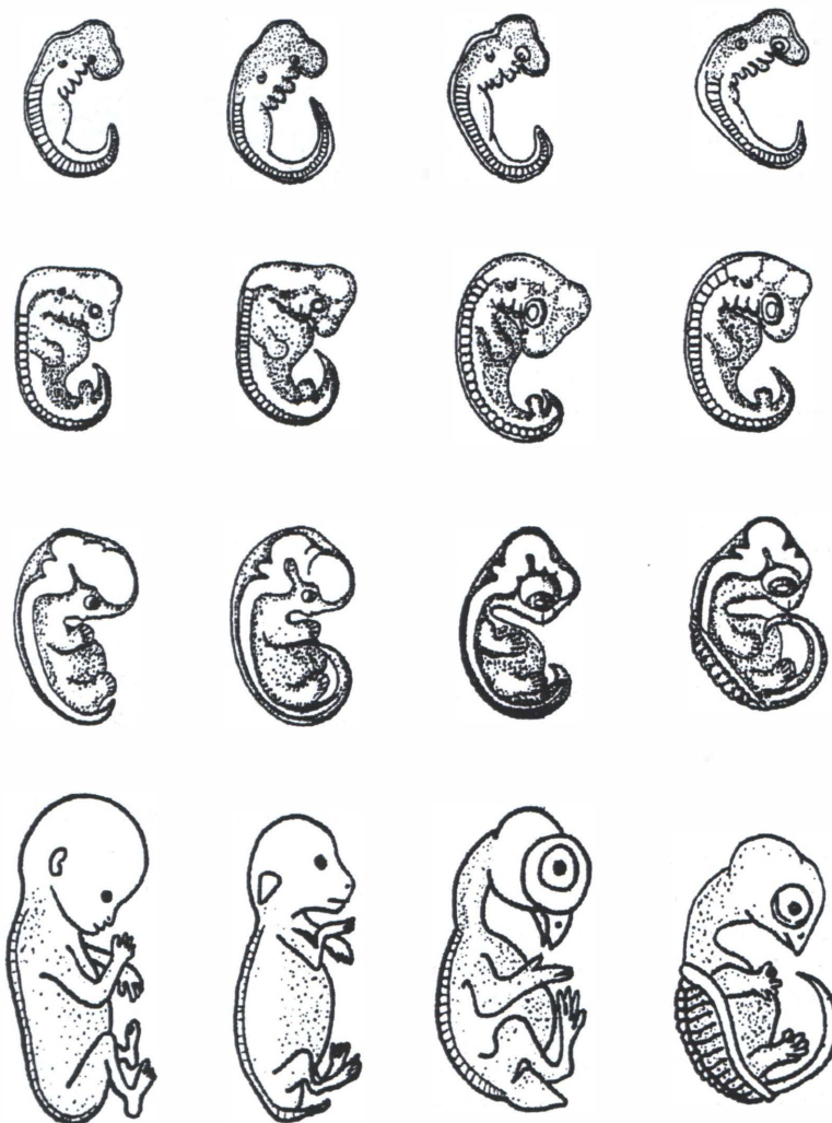
Abb. 2: Entwicklung von Embryonen und Föten in den entsprechenden Stadien bei Vertebraten. Von links nach rechts: Mensch, Kaninchen, Huhn, Schildkröte. Skizze: nach Haeckel von 1868 und 1874; © de Sarre
