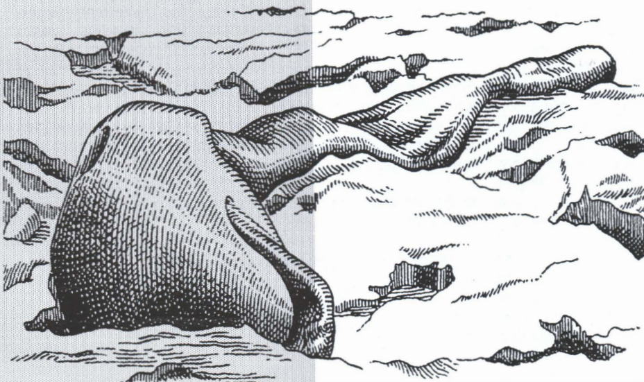
Verunstalteter Entenwal um die Jahrhundertwende (Skizze: Lutz E. Müller)
